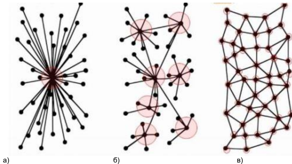
Рисунок 1. Сетевые структуры взаимосвязей пользователей в различных системах: а) централизованные системы; б) блокчейн; в) одноранговая пиринговая сеть.
