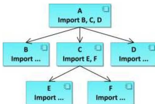
Рис. 1. Пример модульной схемы, модуль А – головной модуль программы
